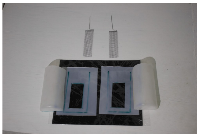
MMO Titan dioksid elektroder og Nafion membran.
